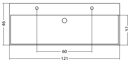
Achteraanzicht
